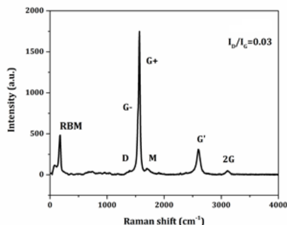
شکل ۴: طیف رامان نمونه نانولوله کربنی تک دیواره فرآوری شده.
