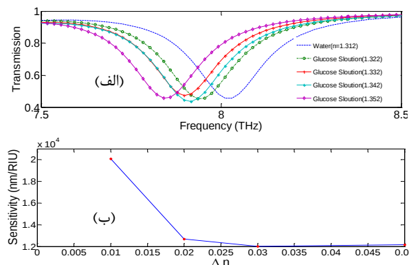
شکل ۶: نمودار (الف) عبور (ب) حساسیت با تغییر ضریب شکست محیط اطراف
