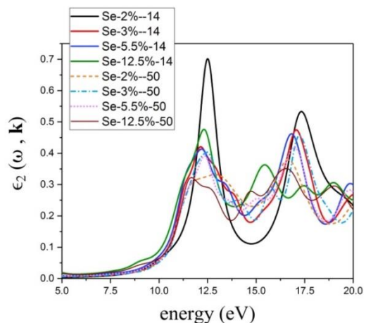
شکل ۶- جزء موهومی دی الکتریک در محدوده فرا بنفش
