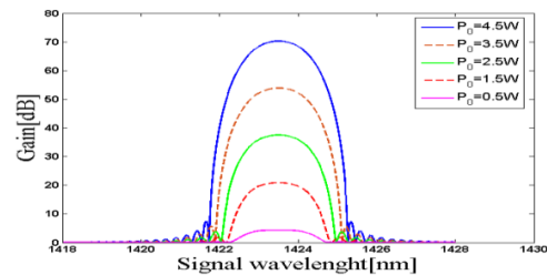
شکل ۴: تغییرات طیف بهره در اثر تغییر توان ورودی در بازه‌ی طول‌موج‌های مختلف سیگنال به ازای \Delta\lambda_m = 1nm و L = 1km و P_0 = 1.5W .
