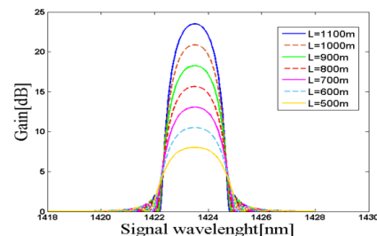
شکل ۵: تغییرات طیف بهره در اثر تغییر طول تار نوری به ازای \Delta\lambda_m = 1nm و P_0 = 1.5W .
