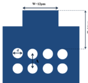
شکل ۱: موجبر سیلیکونی شامل حفره‌های هوا در اطراف مغزی.
