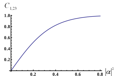
شکل (۱): نمودار سنجۀ توافق حالت |\Psi\rangle بر حسب |\alpha|^2 .
