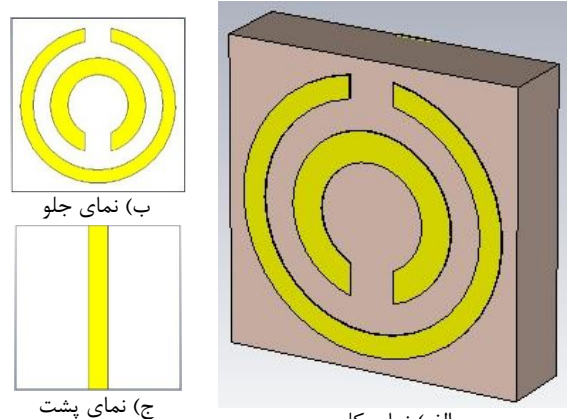
شکل ۱- سلول واحد متشکل از حلقه های دایره ای شکافدار و سیم نازک (الف) نمای کلی سلول (ب) تصویر از جلو (ج) تصویر از پشت
