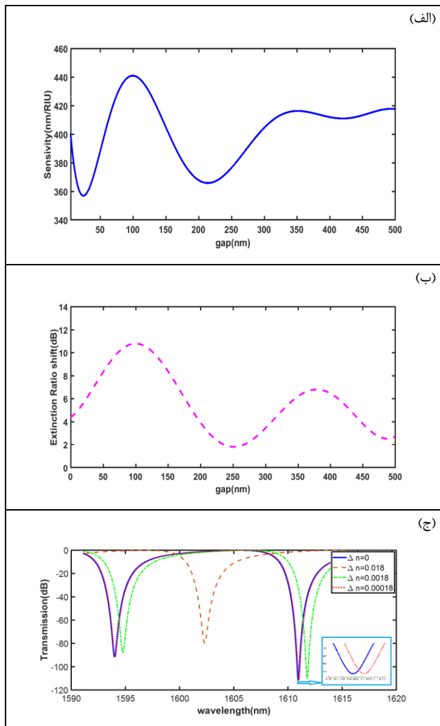
شکل ۲: الف-منحنی حساسیت، ب-منحنی \Delta ER بر حسب تغییر در فاصله، ج- منحنی عبوری بر حسب طول موج که نمودار آبی بدون اعمال تغییرات ضریب شکست و منحنی خط چین قرمز با اعمال \Delta n = 0.018 ، سبز با اعمال \Delta n = 0.0018 و قرمز \Delta n = 0.00018
