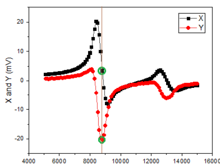
شکل ۳- نمودار تشدید مگنتومتر در فضای باز در بسامد بالا
