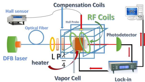
شکل ۱- چیدمان اندازه‌گیری میدان مغناطیسی زمین
