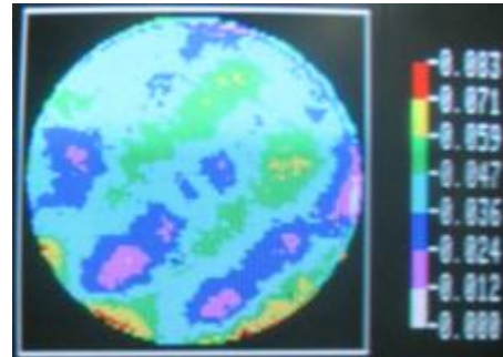
شکل ۸، ناهمواری جبهه‌موج تخت خروجی از مبدل اپتیکی طراحی شده
