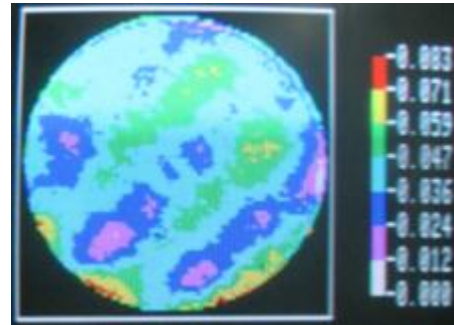
شکل ۸، ناهمبازی جبهه‌موج تخت خروجی از مبدل اپتیکی طراحی شده
