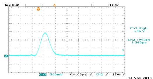
شکل ۴: نمونه هایی از رفتار زمانی جریان تخلیه برای مدار با ۴ لامپ درخش سری. ولتاژ شارژ خازن: بالا) ۱/۴ کیلو ولت، پایین) ۱/۸ کیلو ولت. پهنای زمانی تپ جریان به ترتیب ۴/۱۳ و ۳/۵۴ میکروثانیه و قله جریان تخلیه لامپ ۹۷ و ۱۴۵ آمپر است.
