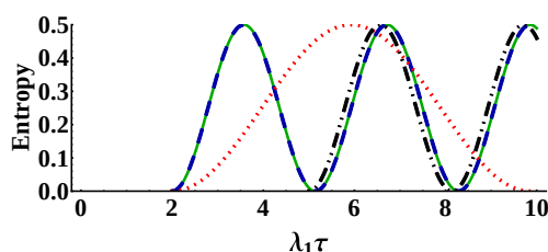
شکل ۳: نمودار آنتروپی برای اتم‌های (۱)، (۸) بر حسب زمان مقیاس‌بندی شده \lambda_1 \tau برای \omega_M / \lambda_1 = 2 ، G / \lambda_1 = 9 (پیوسته سبز)، \omega_M / \lambda_1 = 2 ، G / \lambda_1 = 4 (خط‌چین آبی)، \omega_M / \lambda_1 = 5 ، G / \lambda_1 = 4 (نقطه‌چین قرمز)، \omega_M / \lambda_1 = 2 ، G / \lambda_1 = 4 (خط-نقطه مشکی).
