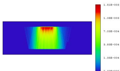
شکل ۲: پروفایل جذب در سطح مقطع تیغه ی لیزر.
