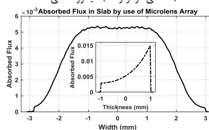
شکل ۸: منحنی دو بعدی جذب در دمش با استفاده از میکروعدسی.
