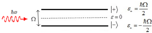
شکل ۱: طرحواره‌ای از سامانه‌ی اتم دو ترازه.
