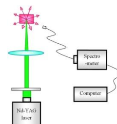
شکل ۱: طرح‌واره‌ای از چیدمان وسایل آزمایش.
