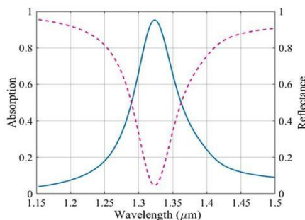
شکل ۲: نمودار طیفی جذب و بازتاب ساختار فلز-دی الکتریک-فلز نانو حسگر پیشنهادی
