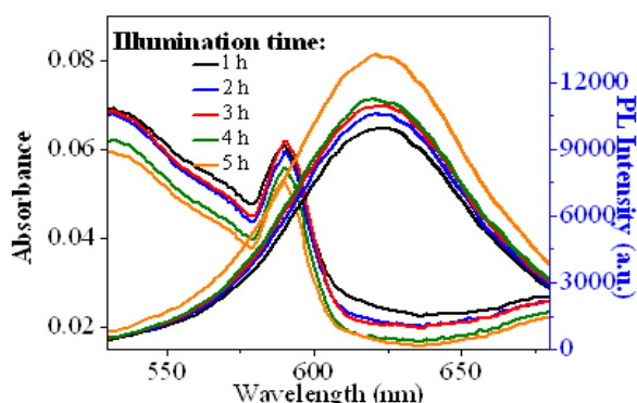
شکل ۲، طیف‌های فلئورسانس و جذب نقاط کوانتومی هسته-پوسته کادمیم تلوراید-کادمیم سولفید برحسب زمان نوردهی
