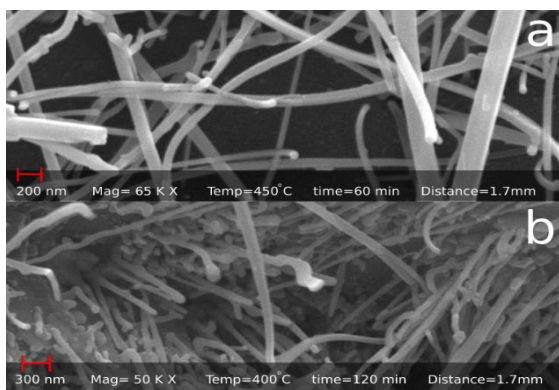
سنتز شده در \text{TeO}_2 مربوط به بهینه ترین سیم های SEM شکل ۳: تصاویر (b) نمای ۴۰۰ درجه (b) نمای ۴۵۰ درجه سلسیوس، زمان ۶۰ دقیقه شرایط سلسیوس، زمان ۱۲۰ دقیقه و در فواصل یکسان ۱/۷ میلیمتری زیر لایه از پودر تلوریوم.
