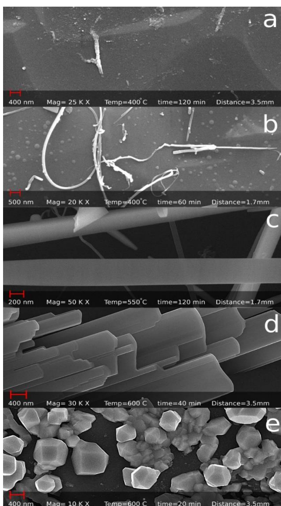
مربوط به تاثیر پارامترها در سنتز نانوسیمها در مقایسه SEM شکل ۴: تصاویر (b) تاثیر تغییر مدت (b) تاثیر تغییر فاصله زیر لایه از پودر تلوریوم با نمونه بهینه (c) تاثیر تغییر دمای تبخیر و (d) و (e) زمان تبخیر
