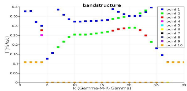
شکل ۱: ساختار نواری تیغه فوتونیک کریستال دو بعدی مثلثی با ضریب شکست 3/34 و دوره تناوب و شعاع حفره به ترتیب 0.46/\mu\text{m} و 0.115/\mu\text{m} میکرومتر و همچنین دارای باند ممنوعه به مرکز حدود 1.556/\mu\text{m} .
