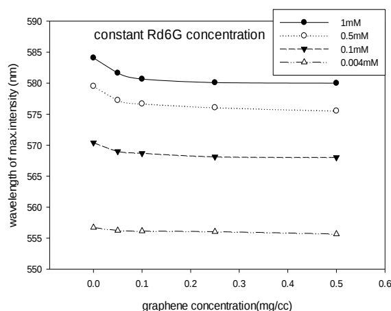
شکل ۳: تاثیر افزایش غلظت گرافن بر طول موج ماکزیمم فلوئورسانس در غلظت های مختلف ردامین
