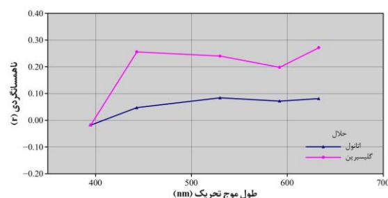
شکل ۳: ناهمسانگردی متیلن‌بلو بر حسب طول‌موج تحریک در باند فلورسانس ۷۰۰ nm
