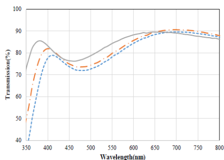
شکل ۳: طیف تراگسیل نمونه شمار ۳ پیش و پس از بازپخت در هوا و خلأ
