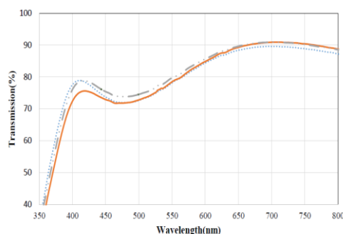
شکل ۲: طیف تراگسیل نمونه‌ها در آهنگ‌های لایه‌نشانی متفاوت
