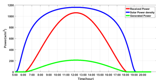
شکل ۵: توان پرتوهای خورشیدی، توان دریافتی و توان تولیدی پنل ثابت برای شهر تهران در تاریخ ۹۴/۰۴/۲۴.
