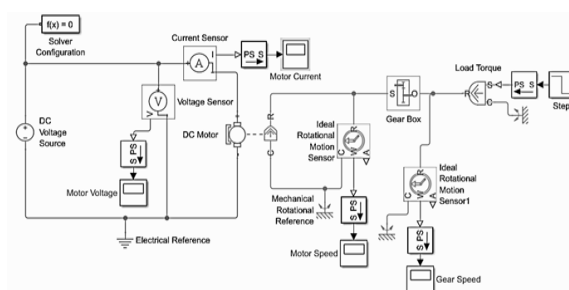
شکل ۳: مدل مورد استفاده در شبیه سازی عملکرد موتور
