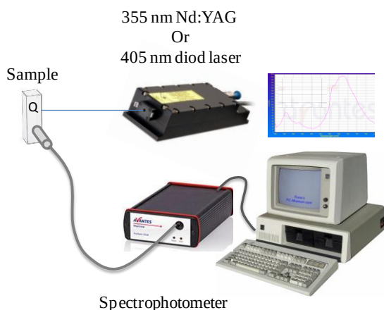
شکل ۱: آرایه آزمایش طیفسنجی فلوئورسانس القایی لیزری محلول کومارین ۴ با طول موجهای ۳۵۵ و ۴۰۵
