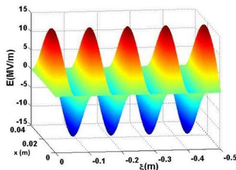
شکل ۴. تغییرات میدان دنباله پالس در موجبر مستطیلی به عرض a = 4 \text{ cm} برای n_0 = 1.24 \times 10^{16} \text{ m}^{-3}
