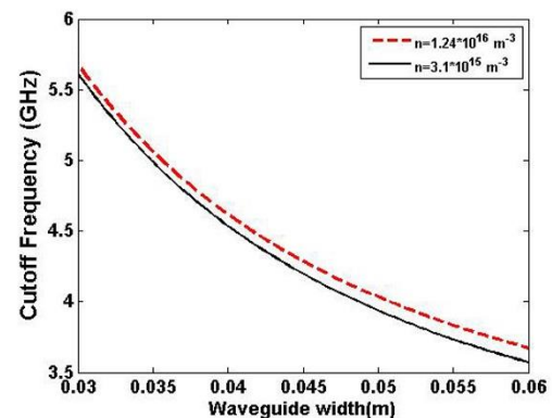
شکل ۱. تغییرات فرکانس قطع موج پلاسمایی بر حسب عرض موجبر برای f = 6 \text{ GHz}
