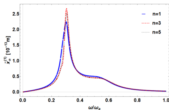
شکل ۵: دامنه جابه‌جایی مرتبه دوم به ازای N = 10 ، d = 2.5r_c و n = 1, 3, 5 ، I = 10^{14} \text{ W/cm}^2 .
