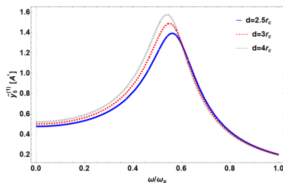
شکل ۴: دامنه جابه‌جایی مرتبه اول به ازای N = 10 ، d = 2.5r_c, 3r_c, 4r_c و I = 10^{14} \text{ W/cm}^2 .
