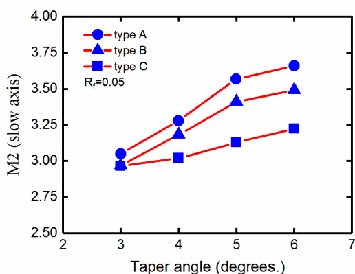
شکل ۴: فاکتور M2 بر حسب زاویه قسمت مخروطی در لیزر دیودهای مخروطی نوع A (دایره)، نوع B (مثلث) و نوع C (مربع) با R_f=0.05 ، W_{\text{ridge}}=3\mu\text{m} و توان خروجی ۱ وات
