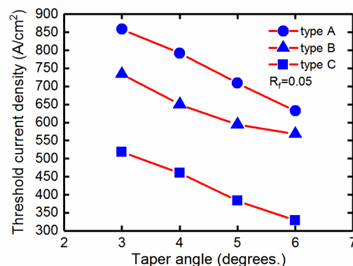
شکل ۵: چگالی جریان آستانه بر حسب زاویه قسمت مخروطی در لیزر دیوهای مخروطی نوع A (دایره)، نوع B (مثلث) و نوع C (مربع) با R_f=0.05 , W_{\text{ridge}}=3\mu\text{m}
