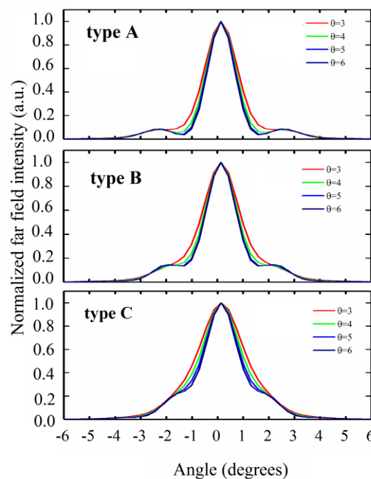
شکل ۳: شدت میدان دور بر حسب زاویه قسمت مخروطی در لیزر دیودهای مخروطی نوع A (دایره)، نوع B (وسط) و نوع C (پایین) با R_f=0.05 ، W_{\text{ridge}}=3\mu\text{m} و توان خروجی ۱ وات
