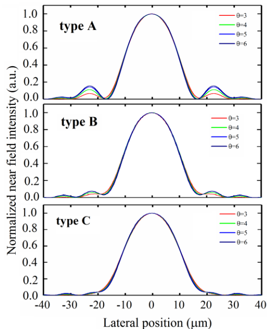
شکل ۲: شدت میدان نزدیک بر حسب مکان در جهت جانبی در لیزر دیودهای مخروطی نوع A (دایره)، نوع B (وسط) و نوع C (پایین) با R_f=0.05 ، W_{\text{ridge}}=3\mu\text{m} و توان خروجی ۱ وات
