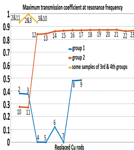
شکل ۵: بیشینه ضریب عبور در جایگذاری میله(های) مسی برای تمامی حالات دسته های اول و دوم و سه حالت از دسته های سوم و چهارم.
