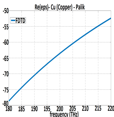
شکل ۶: قسمت حقیقی ضریب دی الکتریک مس از داده های Palik.
