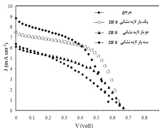
شکل ۵: نمودار جریان-ولتاژ برای سلول خورشیدی پروسکایتی با یک، دو و سه مرتبه لایه‌نشانی ZIF-8 و سلول خورشیدی پروسکایتی مرجع
