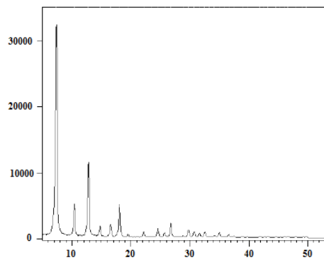
شکل ۲: الگوی XRD برای نانوکریستال‌های ZIF-8
