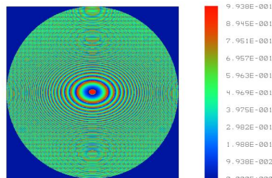
شکل ۴: صفحه‌ی فاز جبران کننده‌ی ابیراهی لنز نمونه برای زاویه‌ی ۱۰ درجه و طول موج آبی به پیمانه‌ی یک طول موج. فاز برحسب یک طول موج معادل 2\pi رادیان بیان شده است.
