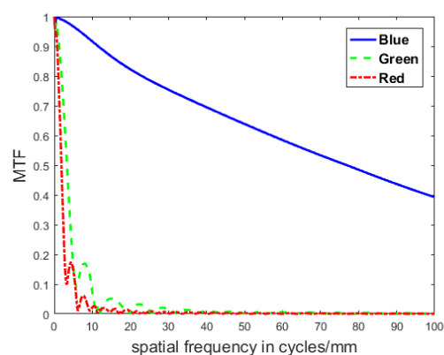
شکل ۵: نمودار MTF برای سه رنگ، وقتی که جبران‌سازی زاویه‌ی ۱۰ درجه تنها برای رنگ آبی انجام شده است.
