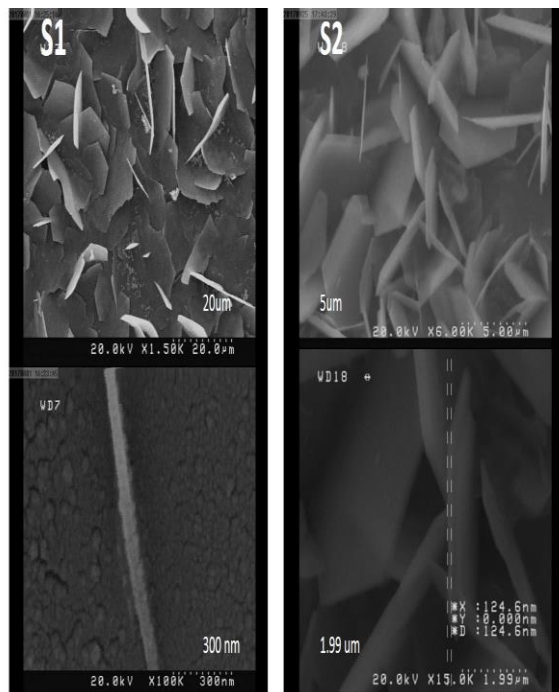
شکل ۱: تصاویر FESEM نانو صفحات اکسید روی
