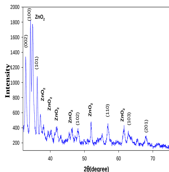
شکل ۲ : نمودار XRD نانو صفحات اکسید روی.
