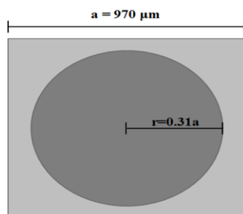
شکل ۱: نمای کناری از سلول واحد بلوری فونونی دو بعدی طراحی شده تنگستن/اپاکسی.
