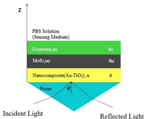
شکل ۱: تصویر شماتیک از ساختار پیشنهادی بیوسنسور نوری مبتنی بر تشدید پلاسمون سطحی حاوی لایه های نانوکامپوزیت، \text{MoS}_2 و گرافن.
