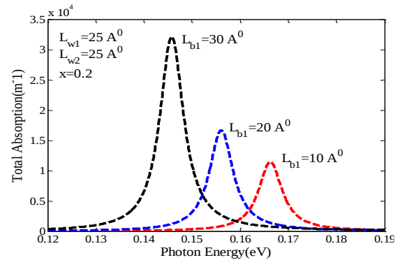
شکل ۲: ضریب جذب نوری کل بر حسب انرژی فوتون فرودی برای مقادیر مختلف پهنای سد.
