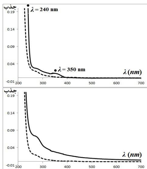
شکل ۳: طیف جذبی UV-Vis از محلول کلرید سدیم بعد از الکترولیز پلاسما، شکل بالا، و بعد از الکترولیز معمولی، شکل پایین. نمودار نقطه چین مربوط به طیف جذبی محلول کلرید سدیم قبل از الکترولیز می باشد.
