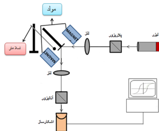
شکل ۶: چیدمان اثر مگنتروپیتیکی کر.
