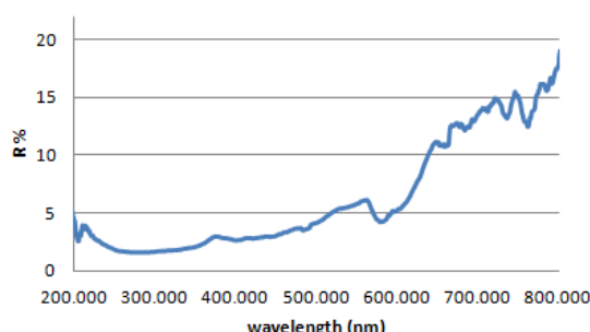
شکل ۴: نمودار بازتاب برحسب طول موج برای قرص ZnO ناخالصی کروم.
