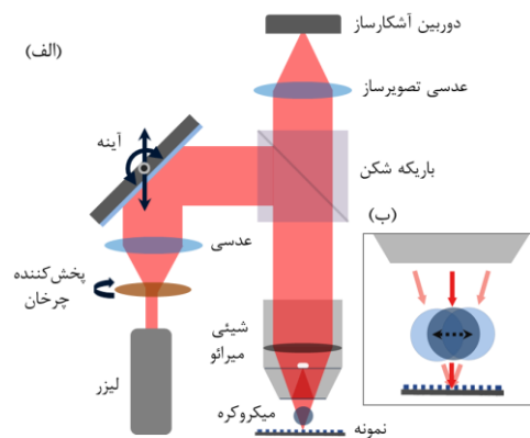
شکل ۱(الف) چیدمان تمامنگاری دیجیتال میرائو با میکروکره تحت نوردهی مایل؛ (ب) تصویر بزرگ‌نمایی‌شده از چیدمان
