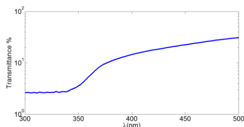
شکل ۲: منحنی طیف عبور برای صفحات اکسید روی.
