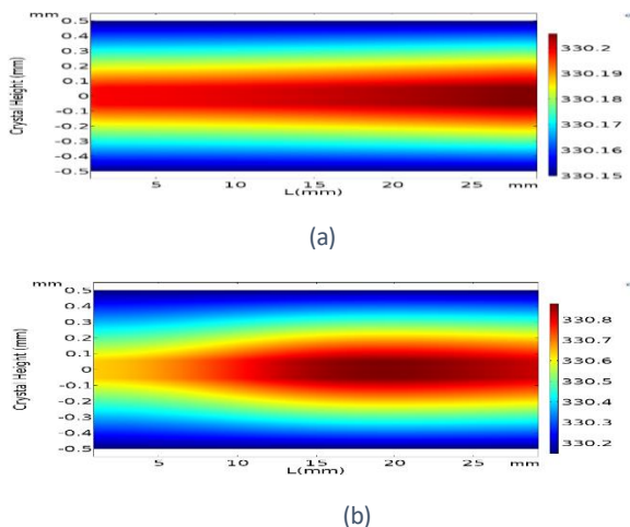
شکل (۱) توزیع حرارتی داخل کریستال MgO:PPSLT به ازای توان فرودی (a) ۵ وات (b) ۵۰ وات
