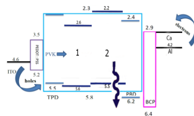
شکل ۶: ساختار دیود نور گسیل آلی و تراز های انرژی آن
