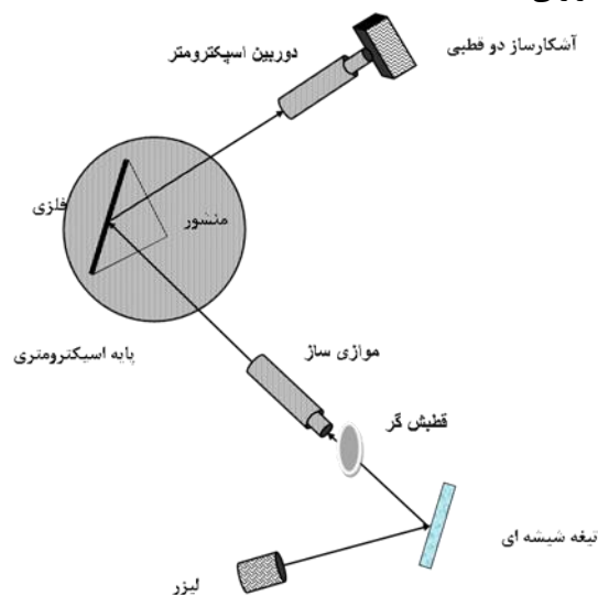
شکل ۱: چیدمان آزمایشگاهی جابجایی گوس- هانچن
