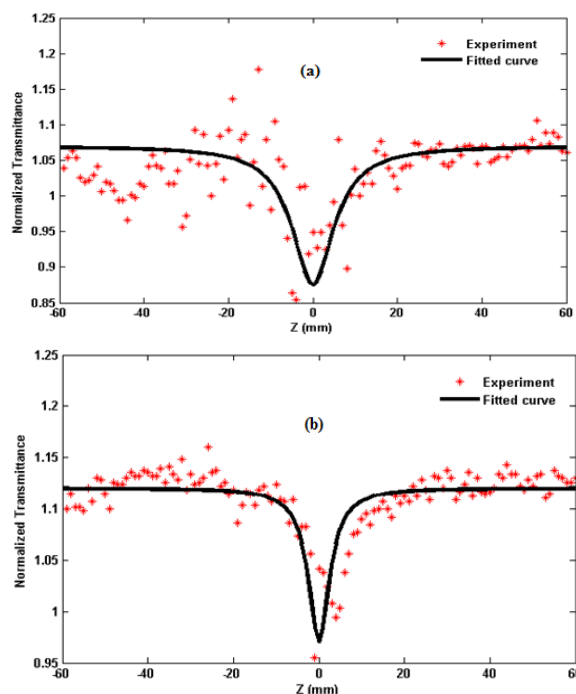
شکل ۴. منحنی جاروب-Z روزنه باز (a) زعفران و (b) چای ترش با شدت 75.0 \text{ kw/m}^2
