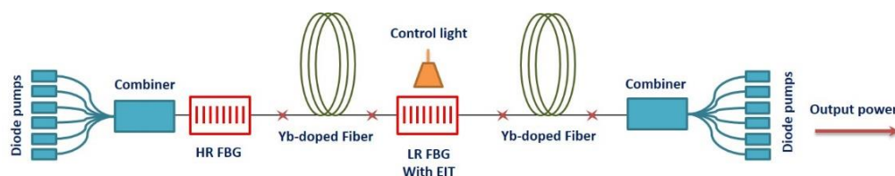
شکل ۱: نمای از MOFPA بر مبنای FBG-EIT
