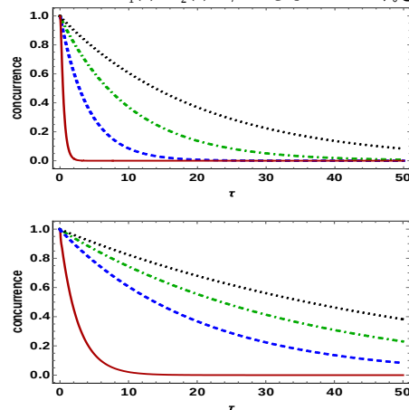
شکل ۲: کمیت تلاقی برحسب \tau = \gamma_0 t در محیط مشترک برای بسامدهای رابی متفاوت به ازای \Delta = 0 (شکل بالا) و به ازای \Delta = 20\gamma_0 (شکل پایین). \Omega = 0 (خط پیوسته)، \Omega = 5\gamma_0 (خط چین)، \Omega = 10\gamma_0 (نقطه-خط) و \Omega = 15\gamma_0 (نقطه-چین) در یک محیط مارکوفی \lambda = 10\gamma_0 با فرض c_1(0) = c_2(0) = 1/\sqrt{2} .
