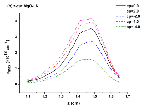
شکل ۲: تغییرات توزیع چگالی پلاسما در محور انتشار به ازای پالسهای لیزری فمتوثانیه با مقدار چیرپ فرکانسی مختلف و با انرژی ۵ میکروژول و طول پالس ۲۵۰ فمتوثانیه کانونی شده داخل کریستال لیتیم نیوبات با (a) برش X و (b) برش Z
