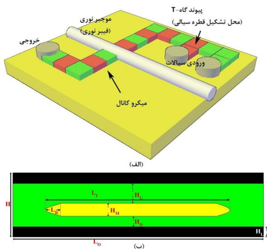
شکل ۱- الف. شمای سه بعدی از طرح را نشان می‌دهد و ب. ساختار دو بعدی از داخل فیبر نوری با شکاف ایجاد شده جهت استفاده از مکانیسم تداخل ماخ زرنر را نشان می‌دهد (مقدار پارامترهای نشان داده شده، L_0=14\mu\text{m} , L_f=10\mu\text{m} , L_R=1\mu\text{m} , H=3\mu\text{m} , H_M=0.5\mu\text{m} , H_U=1\mu\text{m} ، شده، H_0=0.5\mu\text{m} , H_L=0.5\mu\text{m} می‌باشد).
