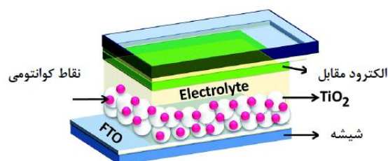
شکل ۱: ساختار سلول‌های خورشیدی حساس شده با نقاط کوانتومی
