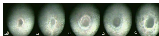
شکل ۷: تصاویر میکروسکوپی حفره‌های ایجاد شده در کندگی لیزری برنج در ۱۵۰۰ پالس و میدان‌های الف) ۰ ولت بر سانتی متر ب) ۵ ولت بر سانتی متر پ) ۱۰ ولت بر سانتی متر ت) ۱۵ ولت بر سانتی متر و ث) ۲۰ ولت بر سانتی متر
