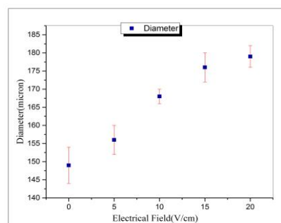
شکل ۸: نمایش تغییرات قطر حفره با افزایش میدان الکتریکی اعمال شده
