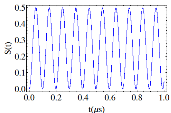
شکل ۲: آنتروپی خطی بر حسب زمان به ازای
