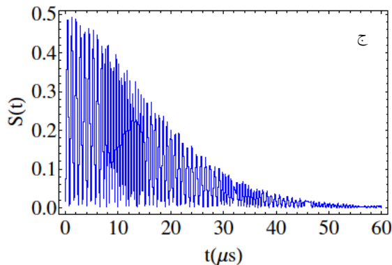
شکل ۳: آنتروپی خطی بر حسب زمان الف ( \kappa = 2\pi \times 50 \text{ kHz} ) ج ( \kappa = 2\pi \times 100 \text{ kHz} ) دیگر پارامترها همانند شکل ۲ در نظر گرفته شده‌اند.
